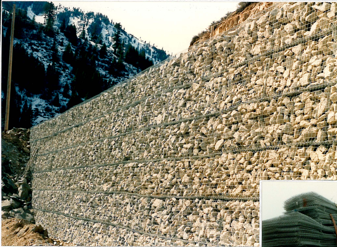
ArtWeld Gabions 9ga.
